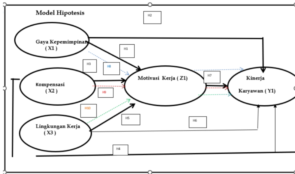
Gambar 1 Kerangka Konseptual
