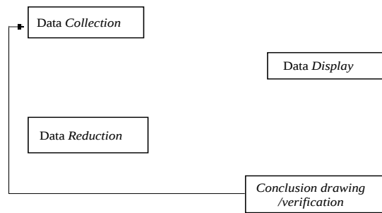
Gambar 2 Analisis data menurut Miles & Huberman
