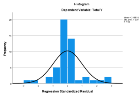
Gambar 1. Histogram Uji Normalitas
