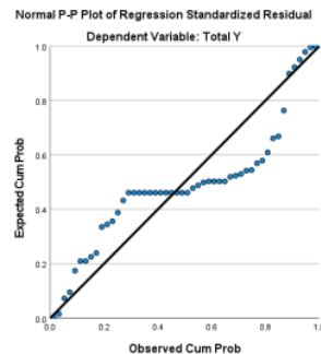
Gambar 2. P-Plot Uji Normalitas
