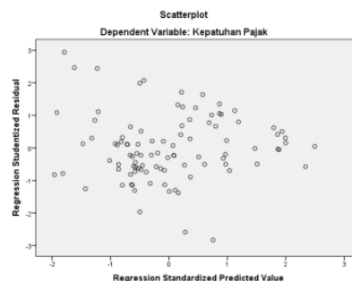
Gambar 4.1 Uji Heteroskedastiditas
